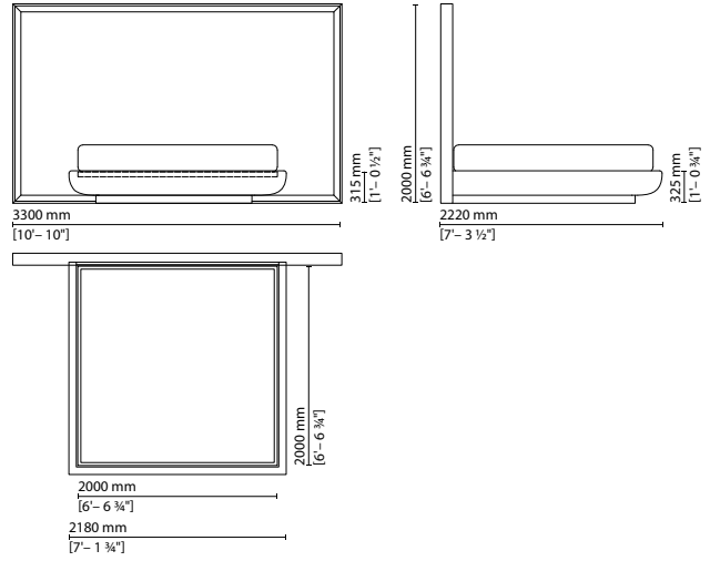
027 403 — Bed 3300×2000 mm (mattress 2000×2000 mm)
