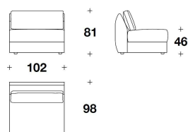
DLS (ECP) ELEMENTO CENTRALE 1 POSTO / 1 SEATER CENTRAL ELEMENT 102x98x81H. - H.S.46cm 40x38 2/3x32H. - H.S.18"
