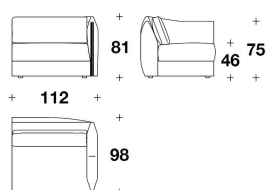
DLS (EPD) - DLS (EPS) ELEMENTO 1 POSTO CON BRACCIOLO DX O SX / 1 SEATER ELEMENT WITH RIGHT OR LEFT ARMREST 112x98x81H. - H.S.46cm 44x38 2/3x32H. - H.S.18"
