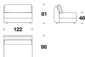
DLS (ECG) BIG : ELEMENTO CENTRALE 1 POSTO / 1 SEATER CENTRAL ELEMENT 122x98x81H. - H.S.46cm 48x38 2/3x32H. - H.S.18"
