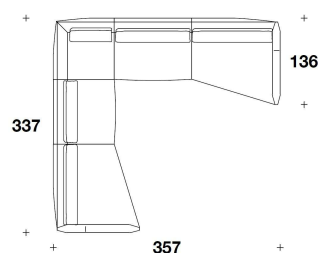
DLS (EOS) + DLS (ECP) + DLS (ANG) + DLS (ECG) + DLS (EOD) H) : ESEMPIO DI COMPOSIZIONE / SECTIONAL SOFA EXAMPLE 357x337x81H. - H.S.46cm 140 1/2x132 2/3x32H. - H.S.18"
