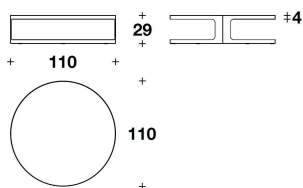
TCV (06) BIG : COFFEE TABLE Ø 110x29H.cm Ø 43 1/3x11 2/4H."
