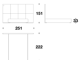
SLE (QUSA) QUEEN USA : LETTO PER MATERASSO / BED FOR MATTRESS 152x205 - 251x222x151H. - H.B.33 cm 60x80 2/3 - 98 2/3x87 1/3x59 1/3H. - H.B.13 "
