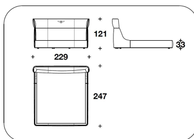
LB1 (KUSA) KING USA : LETTO PER MATERASSO / BED FOR MATTRESS 195x205 - 229x247x121H. - H.B.33cm 76 2/3x80 2/3 - 90x97 1/3x47 2/3H. - H.B.13"
