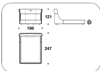
LB1 (QUSA) QUEEN USA : LETTO PER MATERASSO / BED FOR MATTRESS 152x205 - 186x247x121H. - H.B.33cm 60x80 2/3 - 73 1/3x97 1/3x47 2/3H. - H.B.13"
