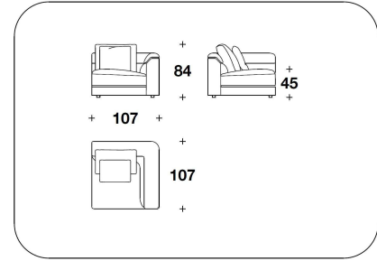
TTN (ANGP) ELEMENTO ANGOLARE / CORNER ELEMENT 107x107x84H. - H.S.45 cm 42x42x33H. - H.S.17 3/4 "
