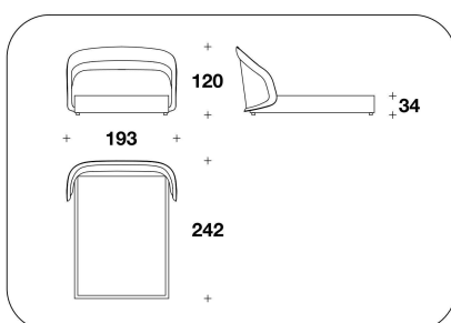
RMG (QUSA) QUEEN USA : LETTO PER MATERASSO / BED FOR MATTRESS 152x205 - 193x242x120H. - H.B.34 cm 60x80 2/3 - 76x95 1/3x47 1/3H. - H.B.13 2/4 "
