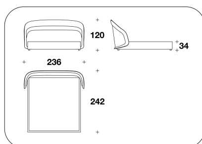
RMG (KUSA) KING USA : LETTO PER MATERASSO / BED FOR MATTRESS 195x205 - 236x242x120H. - H.B.34 cm 76 2/3x80 2/3 - 93x95 1/3x47 1/3H. - H.B.13 2/4 "
